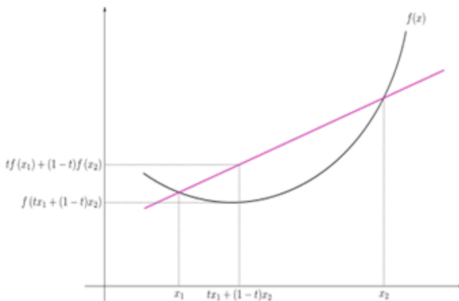
شكل رقم (٣): دالة محدبة الخطر
