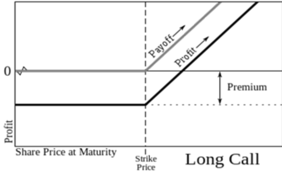
شكل رقم (٧): أرباح مشتري خيار الشراء
