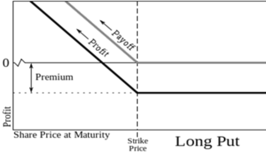
شكل رقم (٨): أرباح مشتري خيار البيع
