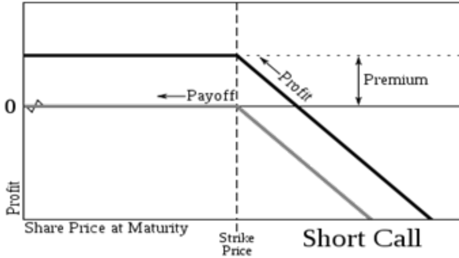
شكل رقم (٩): أرباح بائع خيار الشراء
