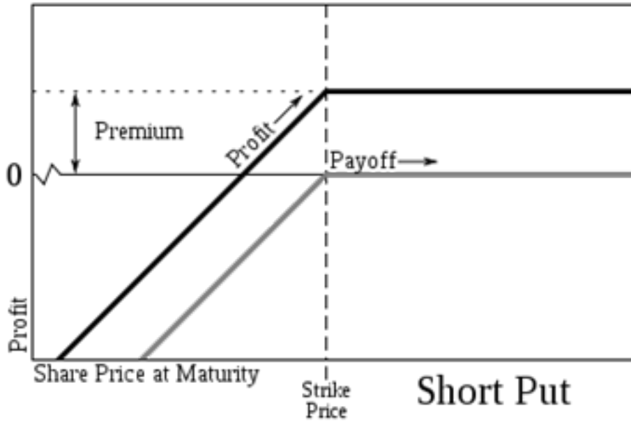
شكل رقم (١٠): أرباح بائع خيار البيع
