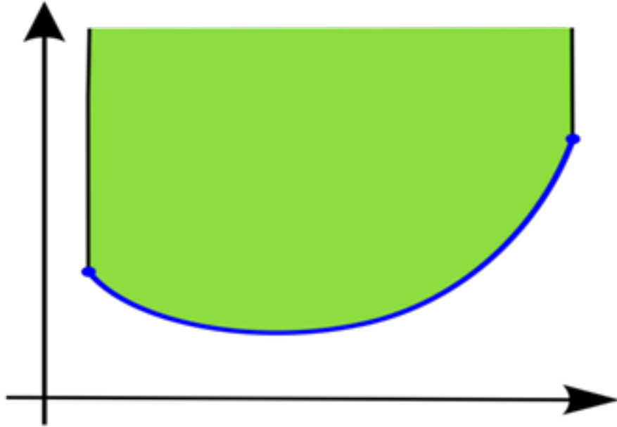
شكل رقم (٥): يعد المنحنى الأزرق، أو الدالة الزرقاء محدبة إذا كان الجزء الأخضر العلوي محدباً
